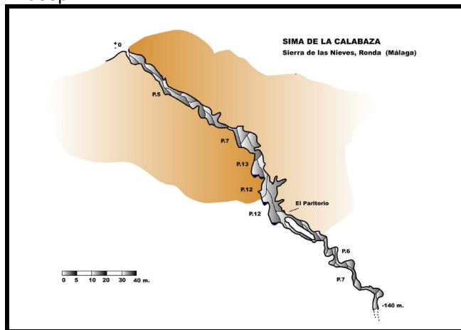
Survey of Sima de la Calabaza after Ces-escarpe.
